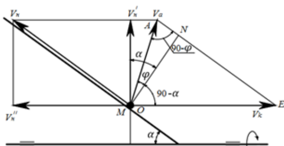
5-расм. Паррак ишчи сиртидаги гўнг бўлагини тезликларининг схемаси
