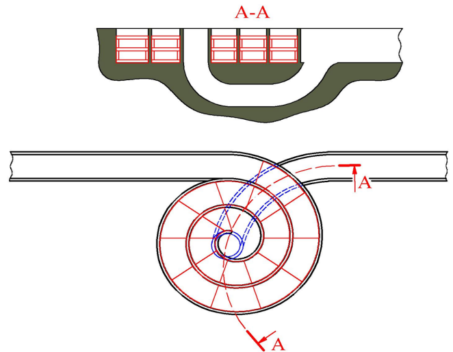
4-rasm. Suv tindirish inshooti buyicha berilgan loyihaning tavsiya etilgan ikkinchi, Arximed spirali asosidagi varianti
