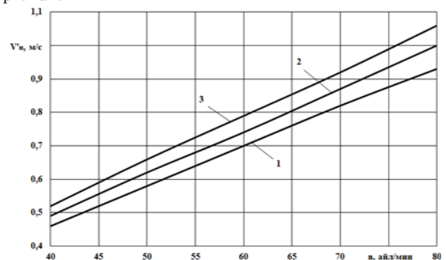
7-расм. Гўнг бўлагини тезлигини парракли шнек айланишлар сонига боғлиқлиқ графиги
