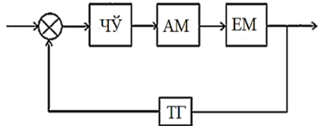
2-расм. Ем майдалаш қурилмаларининг асинхрон моторини частотали бошқаришнинг ёпиқ функционал схемаси: ЧЎ – частота ўзгартгич, АМ – асинхрон мотор, ТГ – тахогенератор, ЕМ – ем майдалаш қурилмаси
