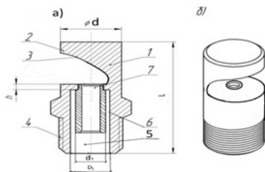
1-расм. Такомиллаштирилган дефлекторли насадка чизмаси ва фотосурати: 1 – корпус; 2 – дефлектор; 3 – экранли юза қайтаргич; 4 – улаш қисми; 5 – марказий канал; 6 – конфузор; 7 – найча.
