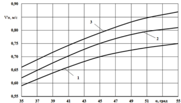
6-расм. Парракдан чиқаётган гўнг бўлагини тезлигини уни ўрнатилиш бурчагига боғлиқлиқ графиги
